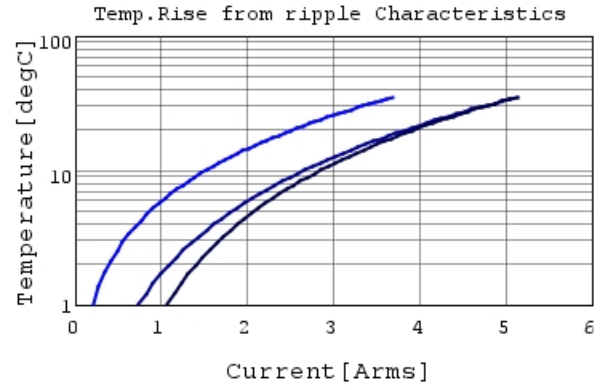
GRM21BR70J106KE76 Temp.rise — 80kHz
